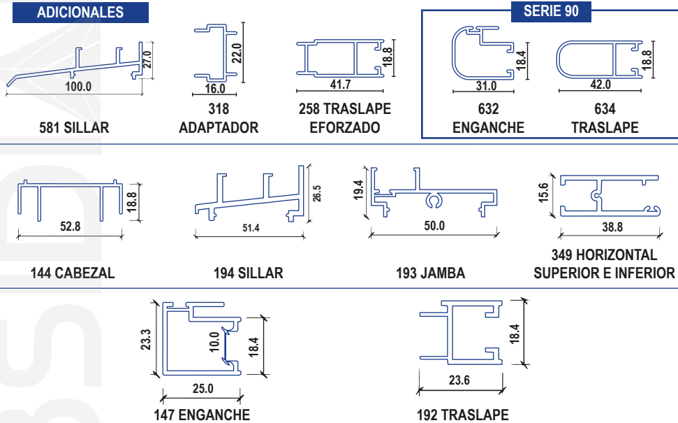
DESPIECE PERFILES VENTANA CORREDIZA 5020 (MARCO CON DOS NAVES UNA FIJA Y UNA CORREDIZA)
