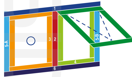
DESPIECE PERFILES VENTANA PROYECTANTE 3831 (MARCO CON UN FIJO Y UNA PROYECTANTE)
