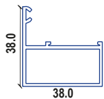
416 ESQUINERO
