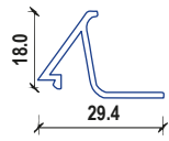
481 PISAVIDRIO 20MM
