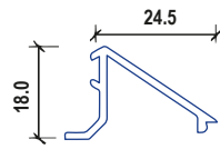
177 PISAVIDRIO
