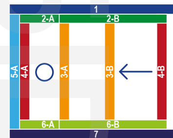
DESPIECE PERFILES VENTANA CORREDIZA 744 (MARCO CON DOS NAVES UNA FIJA Y UNA CORREDIZA)
