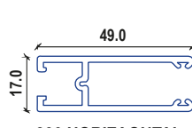
390 HORIZONTAL INFERIOR
