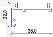
175 ADAPTADOR
