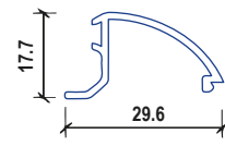
635 PISAVIDRIO
