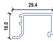
414 PISAVIDRIO CUADRADO
