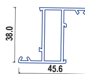
176 MARCO NAVE
